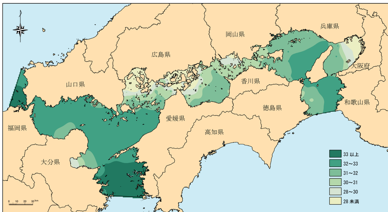
図 4-12 令和4年度 塩分（夏季表層）分布図
