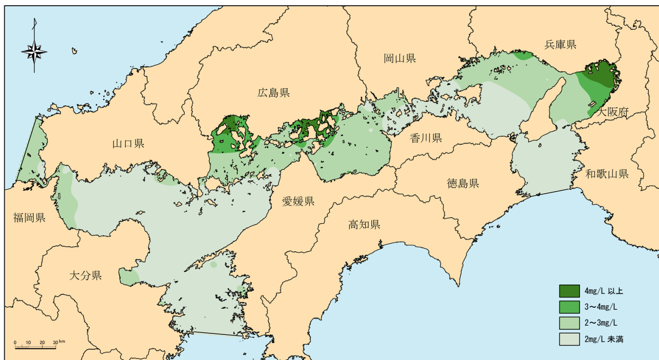
図 4-13 令和4年度 COD（夏季表層）分布図
