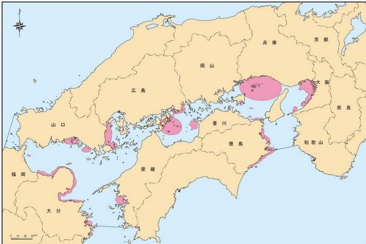
図5-2 赤潮発生海域(令和2年)
