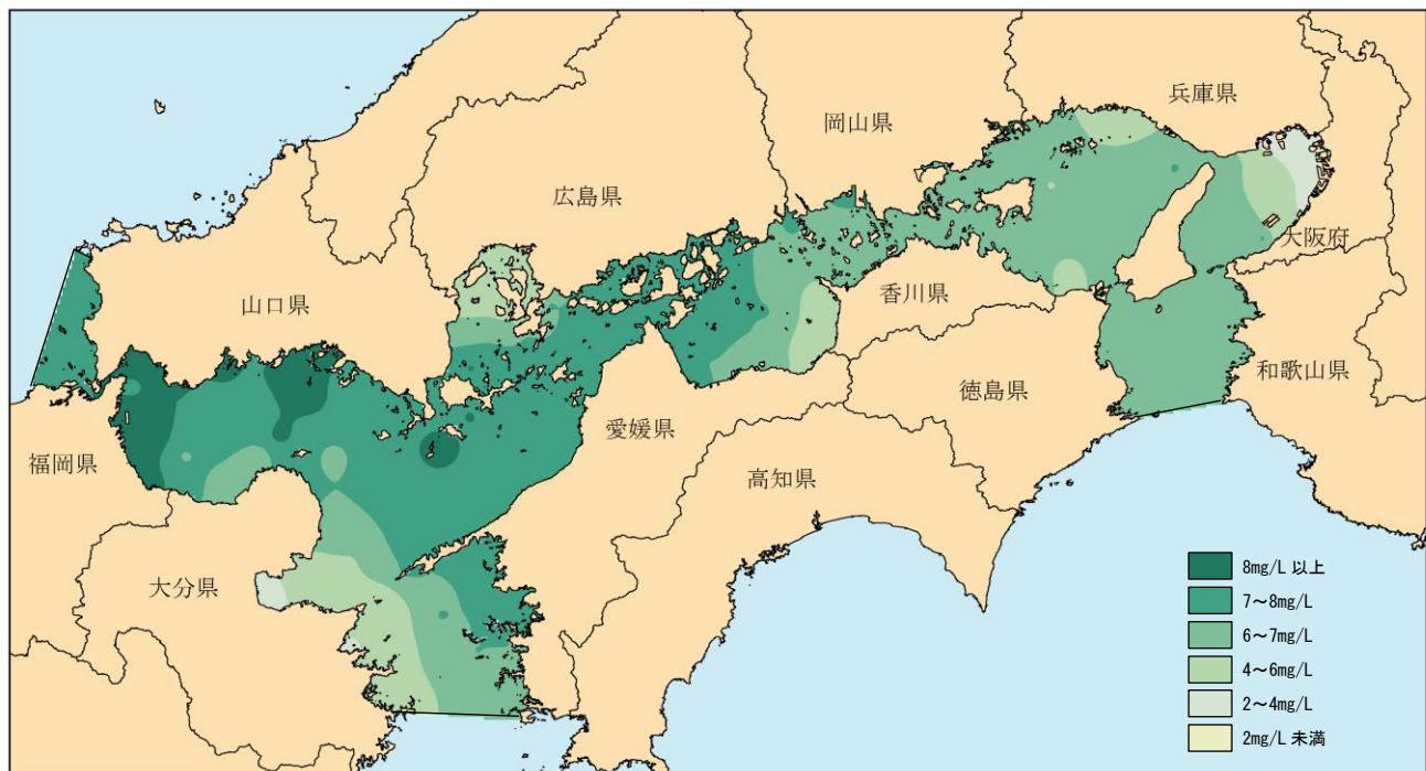
図 4-14 (1) 令和元年度 DO濃度（夏季底層）分布図
