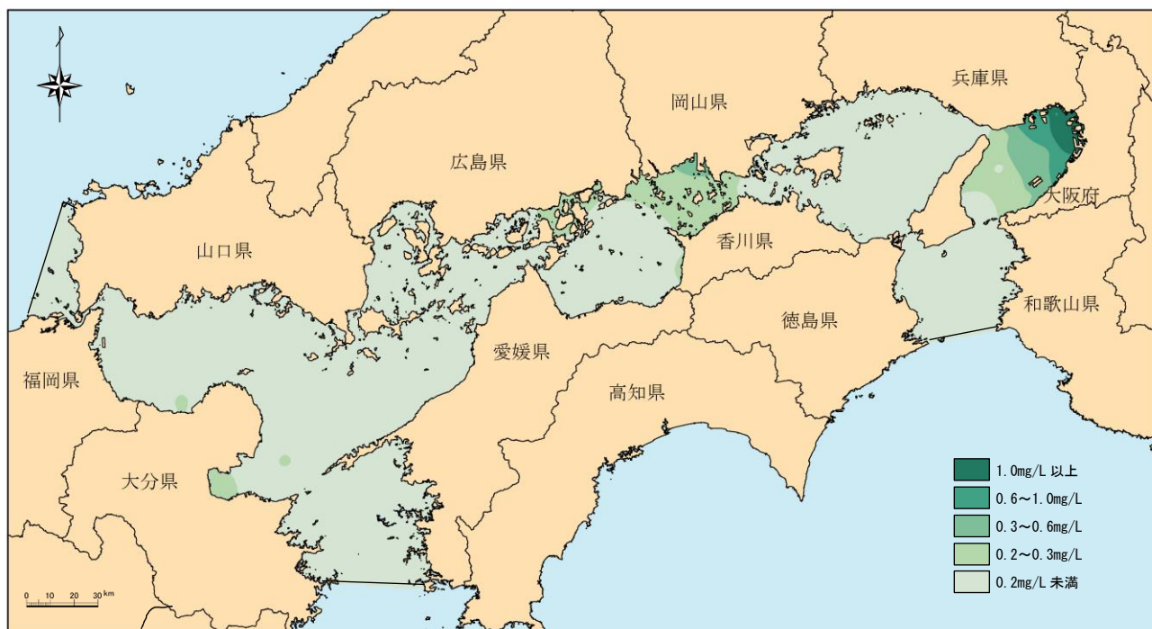
図 4-15 令和元年度 全窒素（夏季表層）分布図
