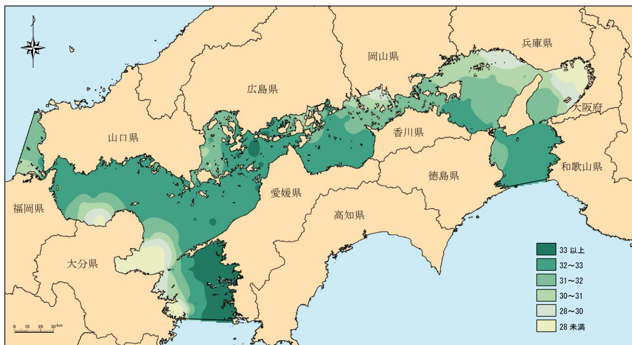
図 4-12 令和元年度 塩分（夏季表層）分布図
