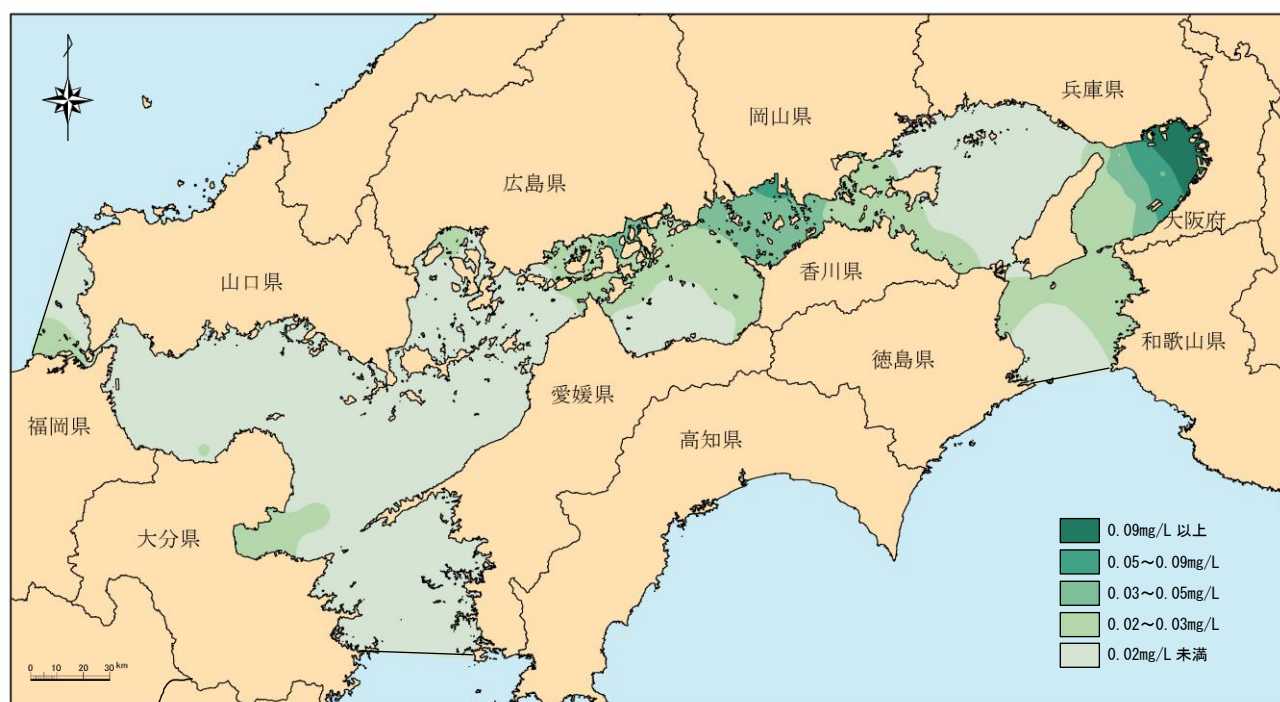
図 4-16 令和元年度 全磷（夏季表層）分布図
