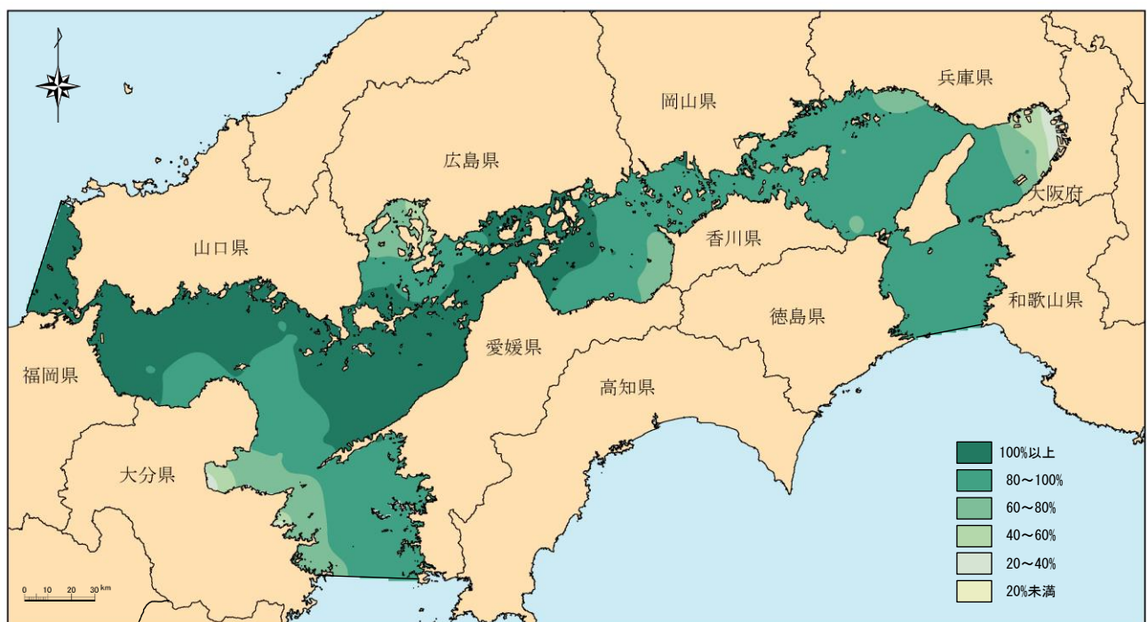
図 4-14 (2) 令和元年度 DO飽和度（夏季底層）分布図
