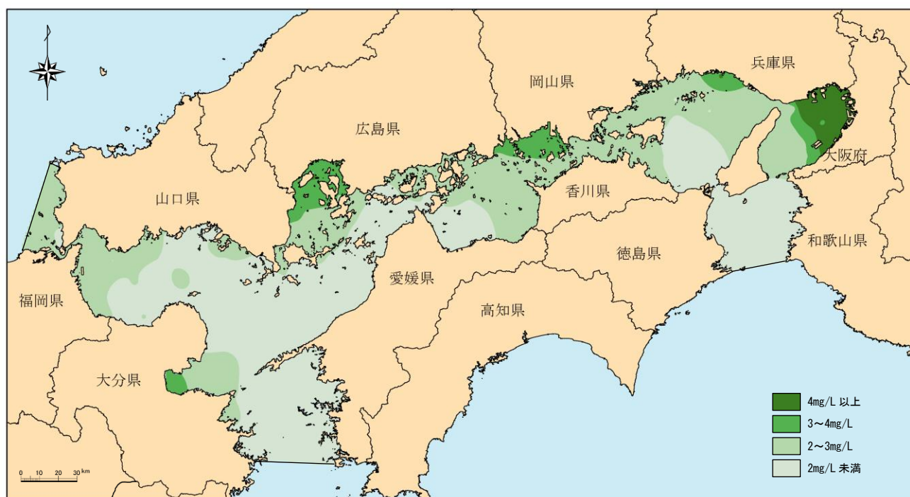
図 4-13 令和元年度 COD（夏季表層）分布図
