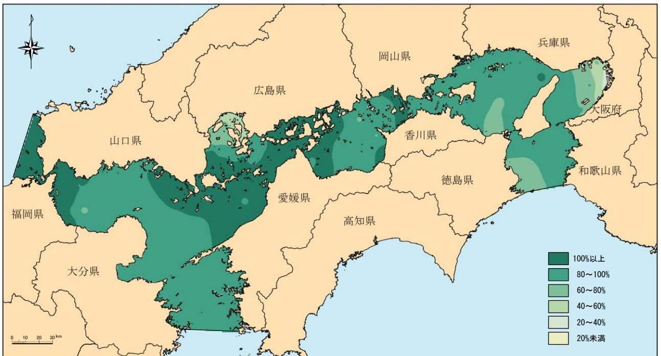
図4-14 (2) 平成30年度 DO飽和度（夏季底層）分布図
