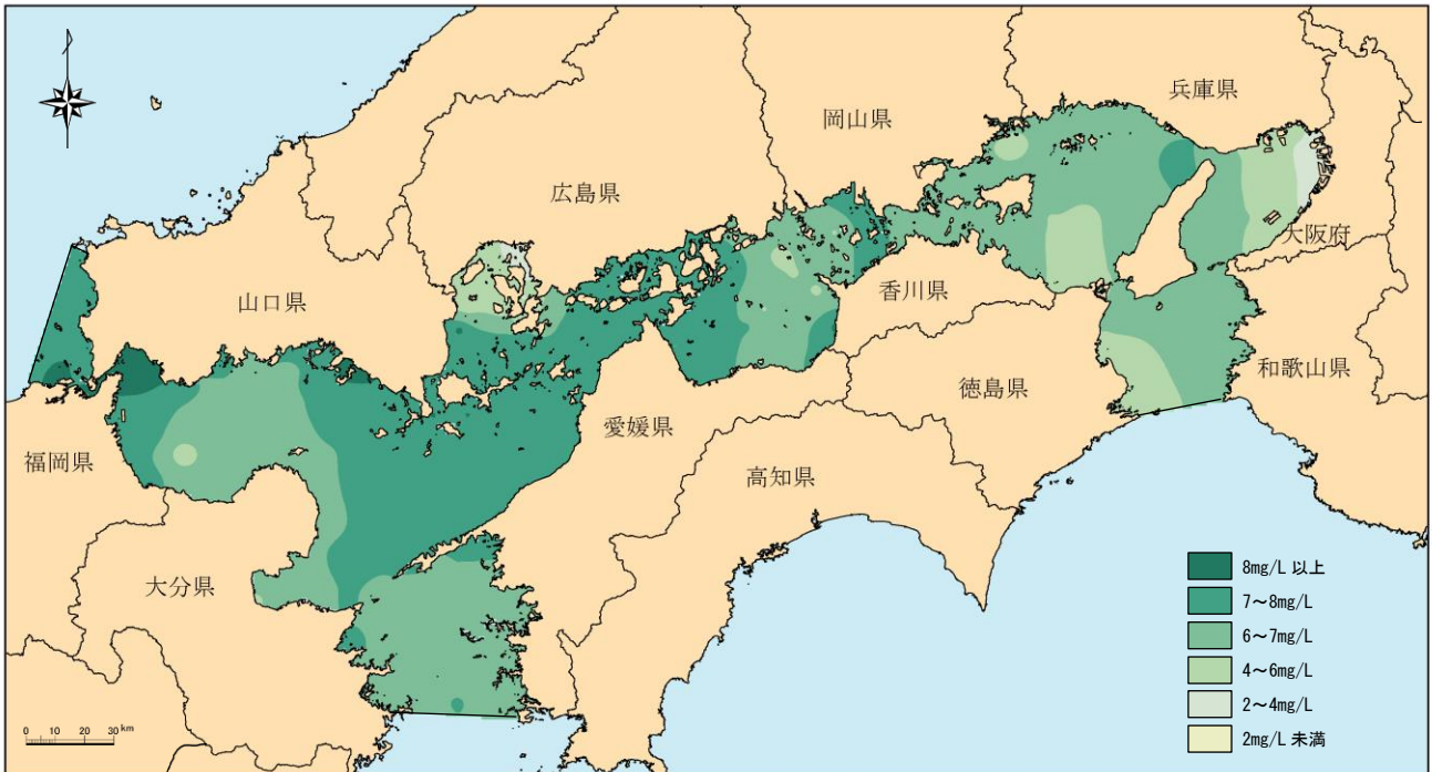
図4-14 (1) 平成30年度 DO濃度（夏季底層）分布図
