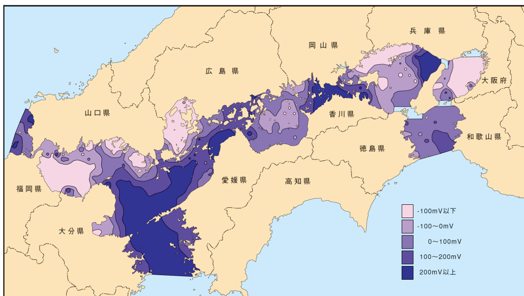
図 4-17 (2) 底質分布図
