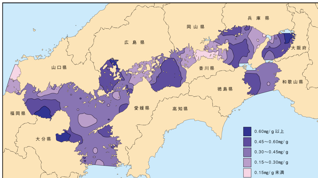
[全磷]
