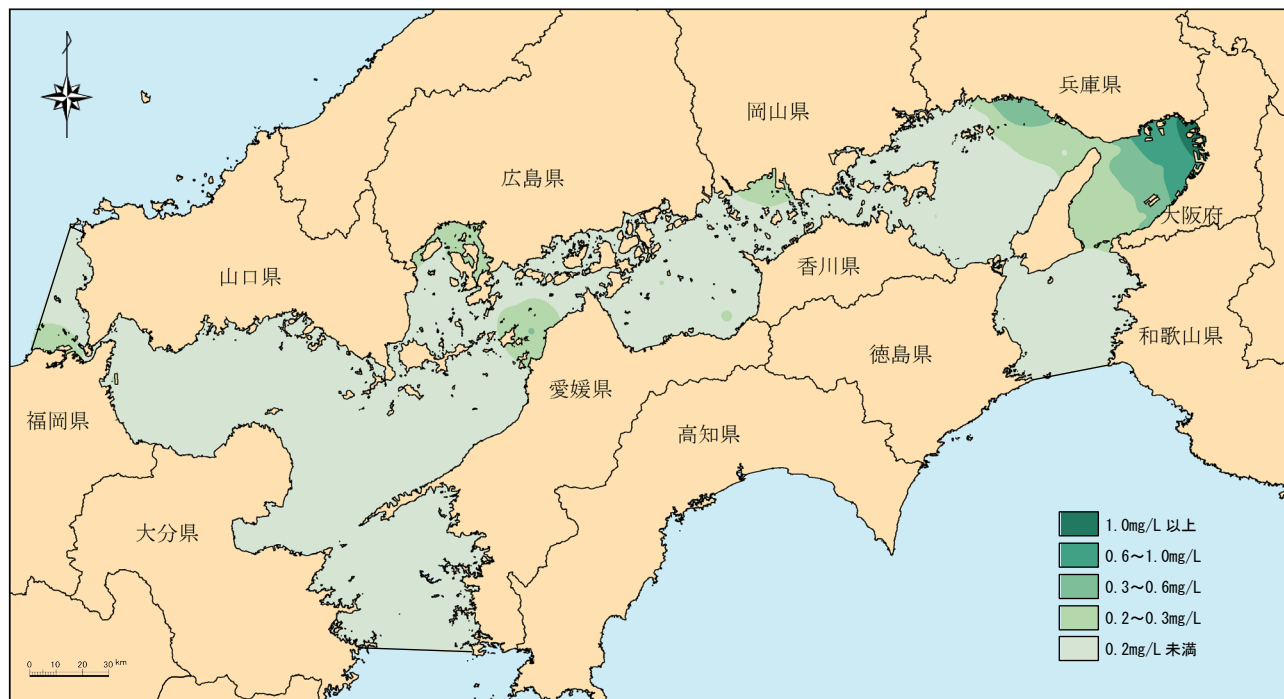
図 4-15 平成 29 年度 全窒素（夏季表層）分布図
