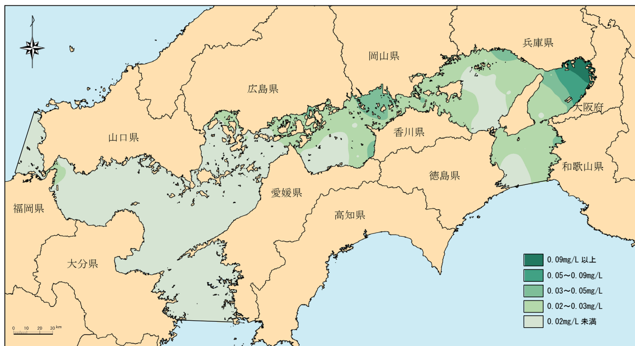
図 4-16 平成 29 年度 全燐（夏季表層）分布図
