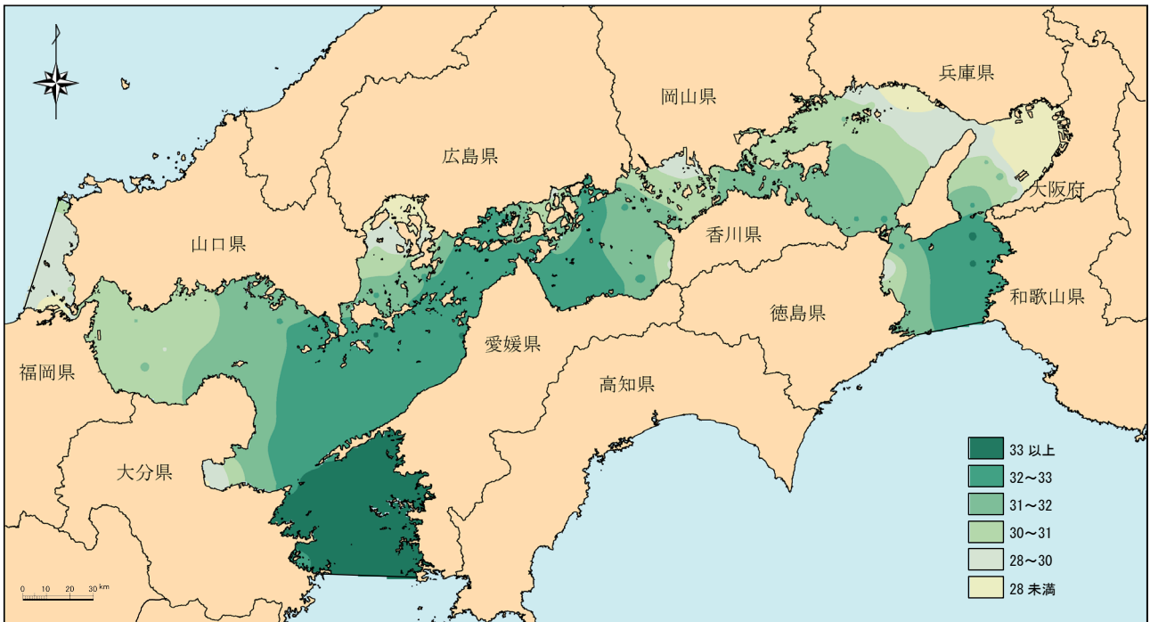
図4-12 平成29年度 塩分（夏季表層）分布図
