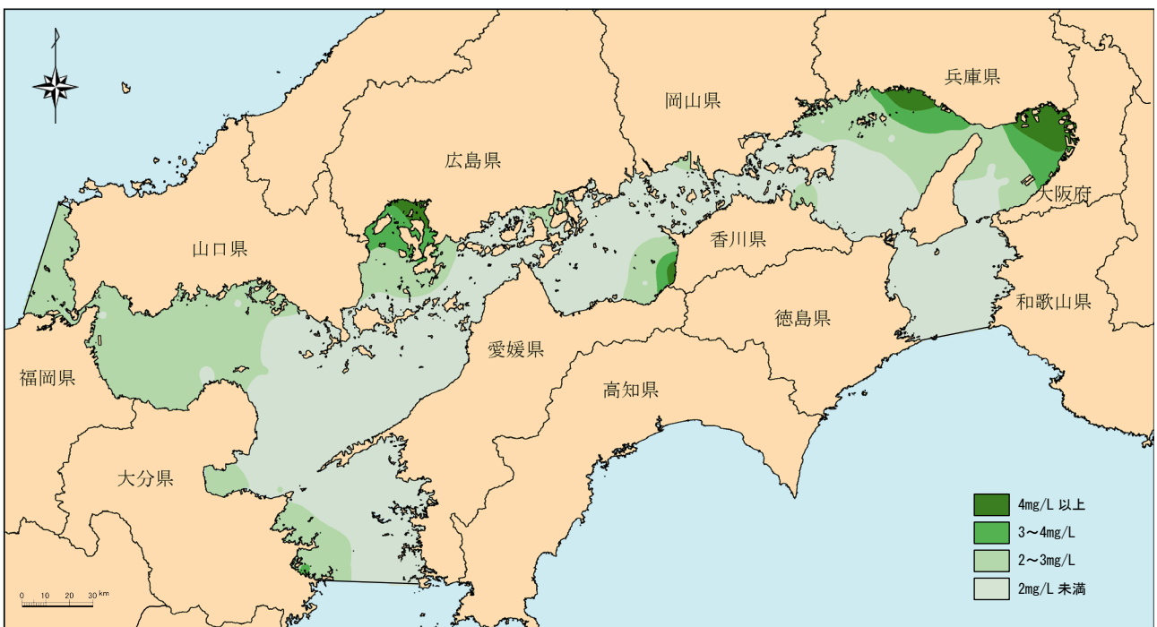
図4-13 平成29年度 COD（夏季表層）分布図
